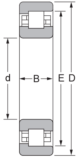
- RJA
