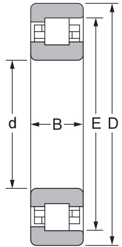
NF
