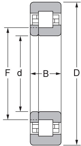
NUP
