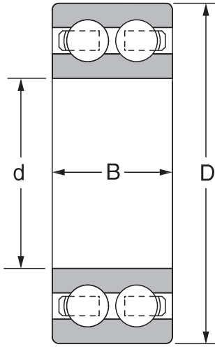
4200B
