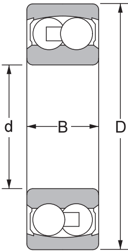
2200 - 2RS 2300 - 2RS
