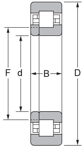
-- RJB
