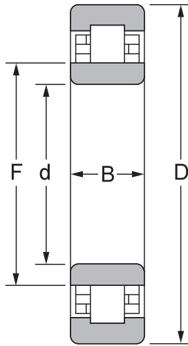
NU
