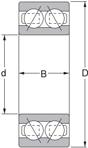
32-B & 33-B 25°
