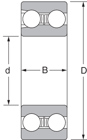
4200M 4300M
